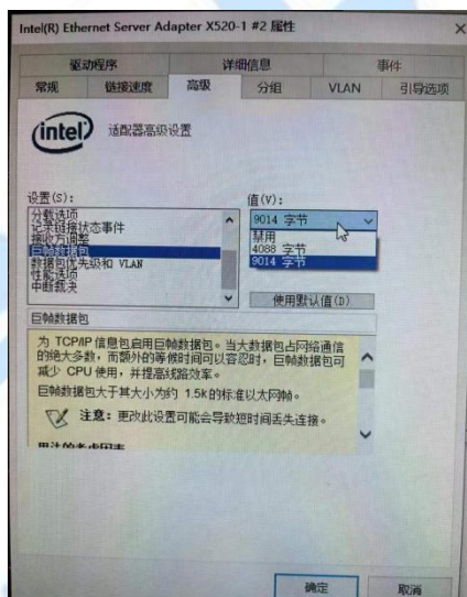
图 3-4 开启网卡巨帧
