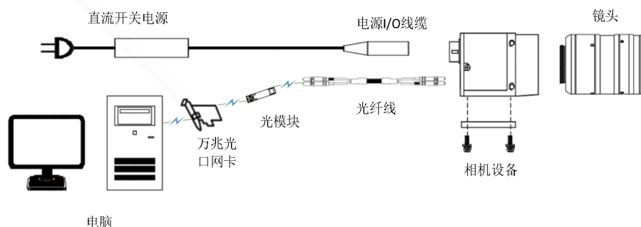
图 3-2 相机整机连接
