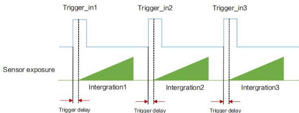
图 4-6 信号延迟原理
