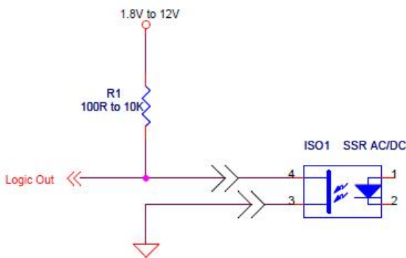
图 2-5 开放排水逻辑驱动器电路
