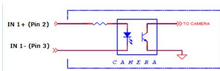
图 2-2 光电隔离输入
