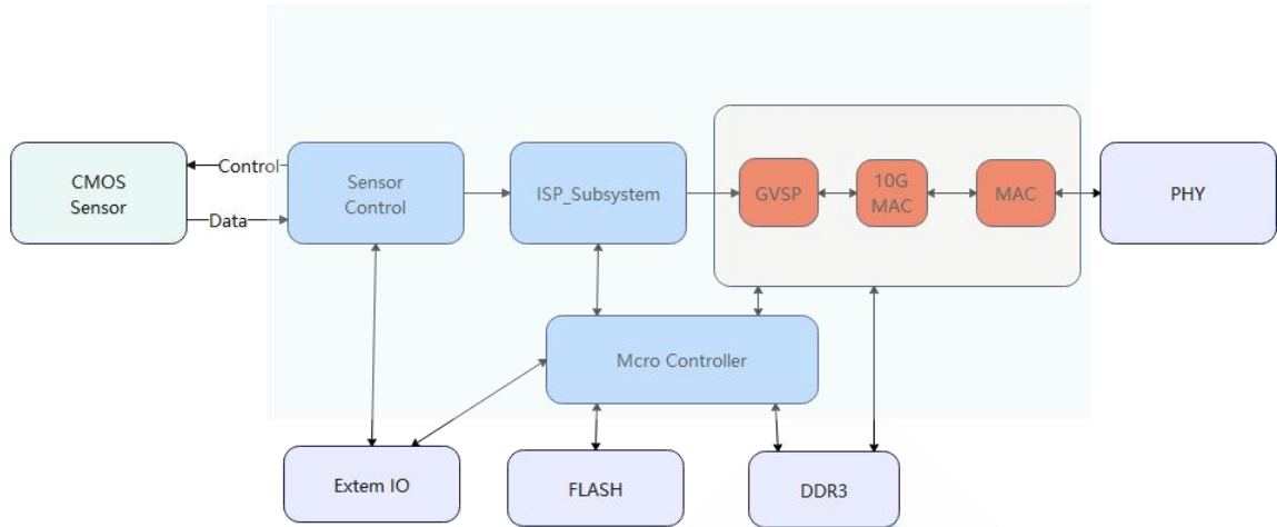
图 1-1 工作原理图
