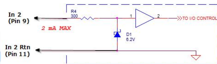
图 2-3 TTL/LVTTL 输入
