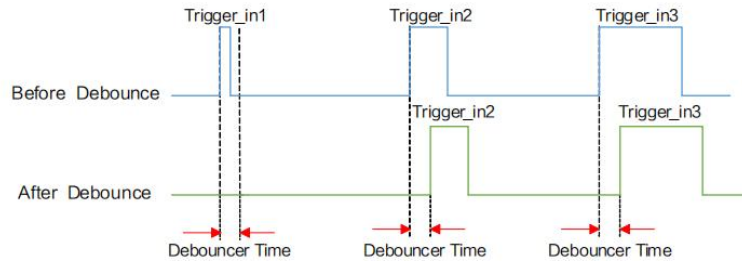
图 4-10 触发防抖时序图
