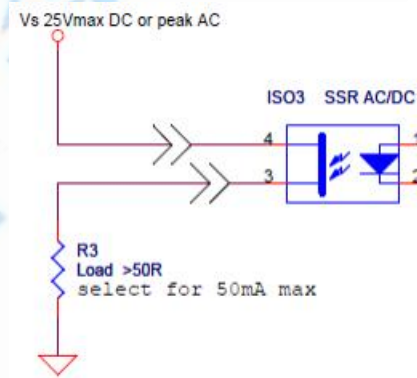
图 2-7 高侧负载驱动器电路
