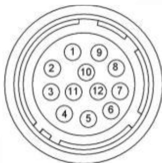
图 2-1 Hirose 连接器
