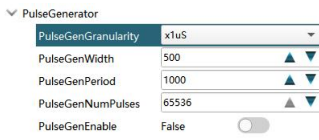
图 4-5 脉冲触发器触发设置
