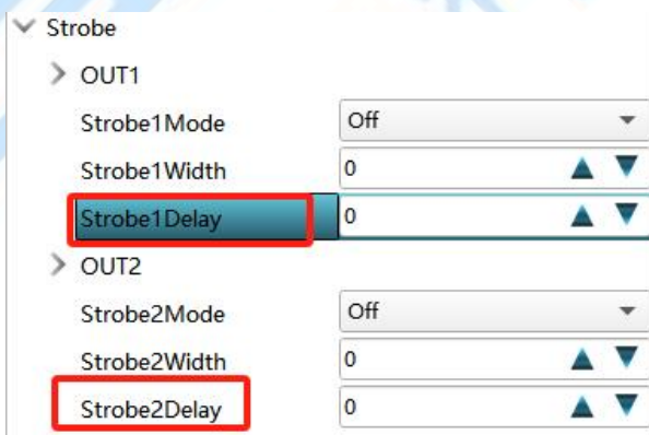
图 4-14 Strobe 输出延迟参数设置
