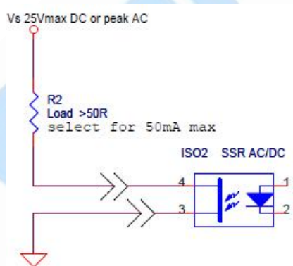
图 2-6 低侧负载驱动器电路
