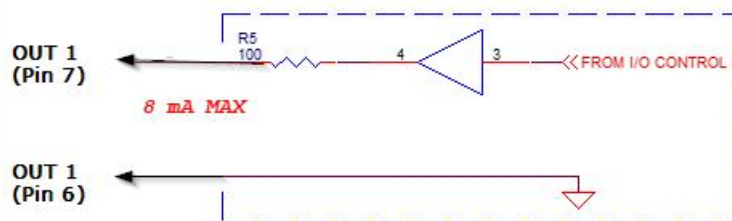
图 3-5 OUT1 LVTTTL 电气连接
