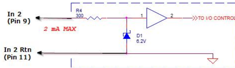
图 3-4 IN2 电气连接
