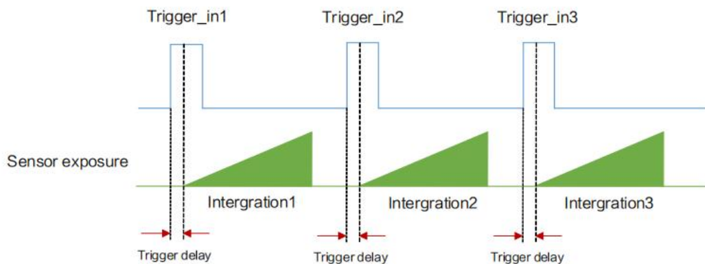
图 5-6 信号延迟原理
