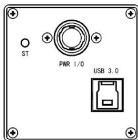
图 3-1 相机部分外观
