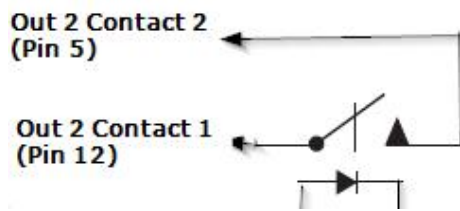
图 3-6 OUT2 光电隔离电气连接
