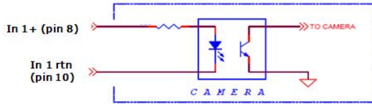
图 3-3 IN1 电气连接
